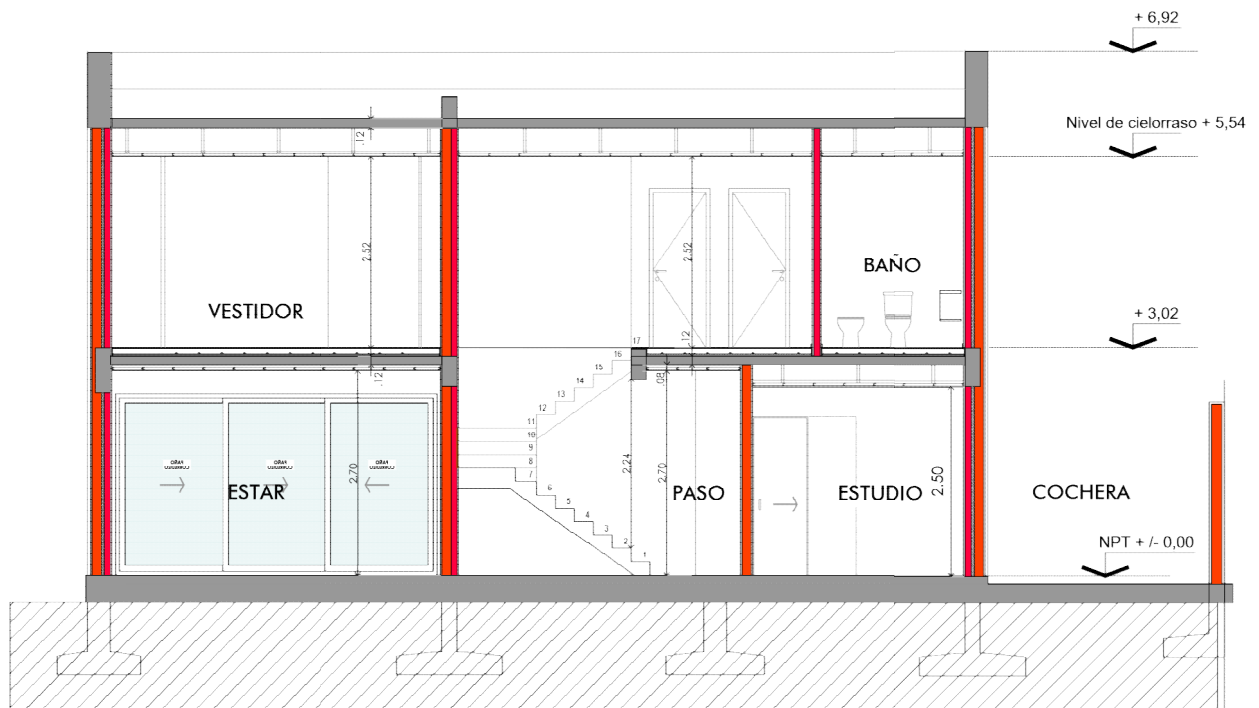
CORTE B-B
