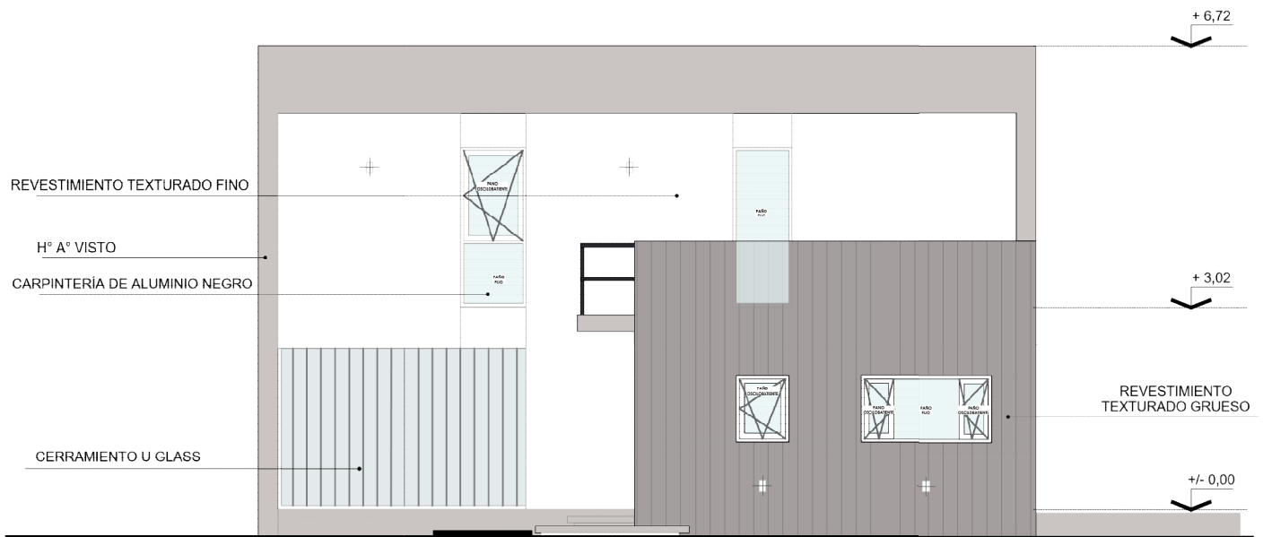
VISTA FRENTE
