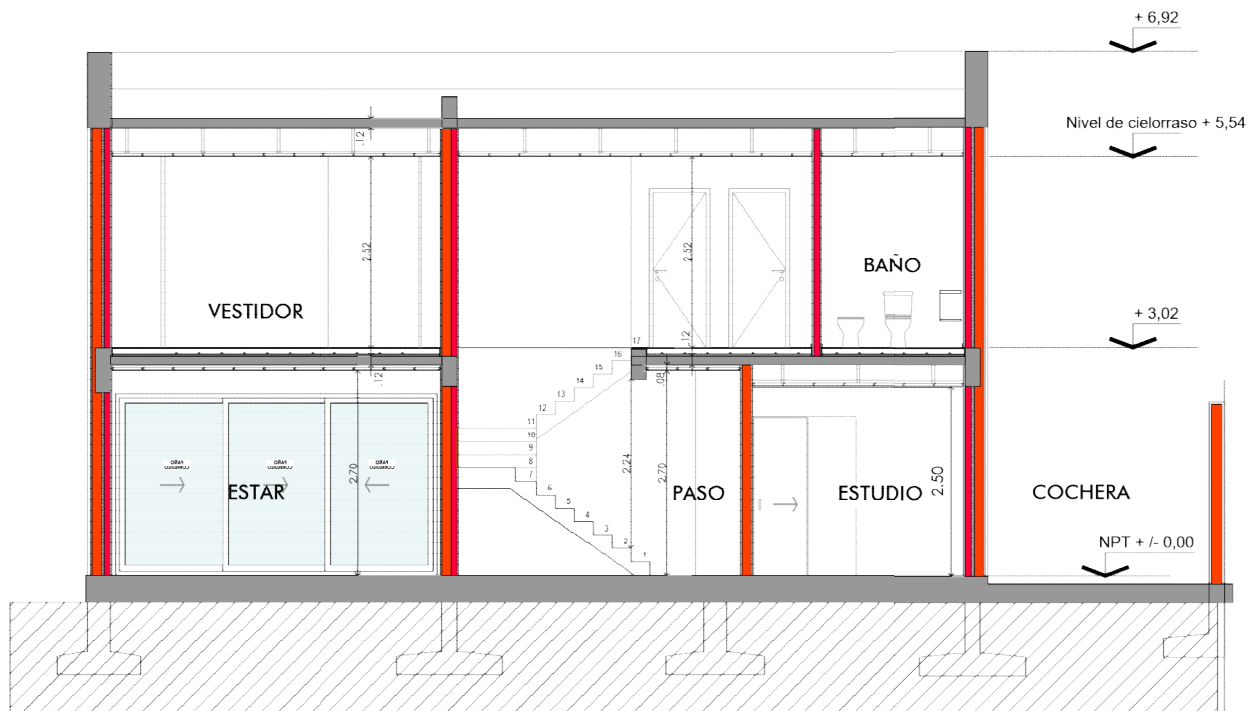
CORTE B-B
